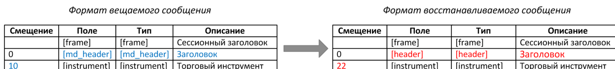
Рисунок 1. Изменение формата сообщения с рыночными данными в шлюзе восстановления
